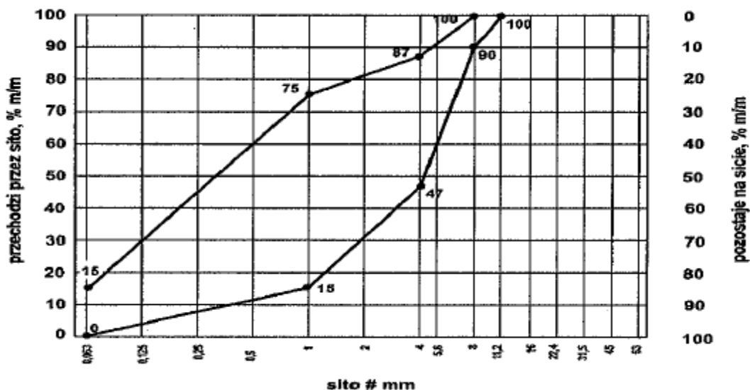
Rys 1. Mieszanka kruszyw 0/8
