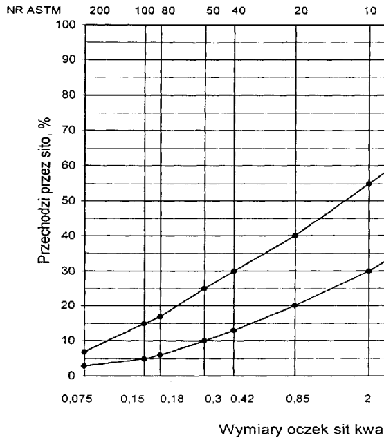
Rys. 8. Krzywe graniczne uziarnienia mieszanki mineralnej BA od 0 do 20 mm do warstwy wiążącej, wyrównawczej i wzmacniającej nawierzchni drogi o obciążeniu ruchem KR1 lub KR2
